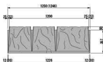
基礎ブロック
