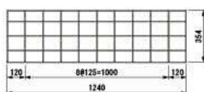
空積用 L 型金網
