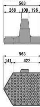
縦半型 右
