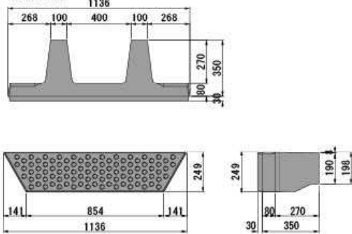
横半天端
