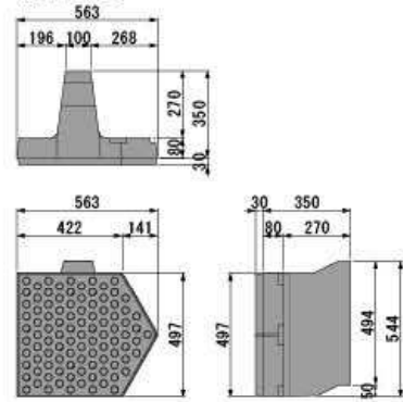
縦半型 左
