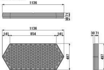
調整パネル
