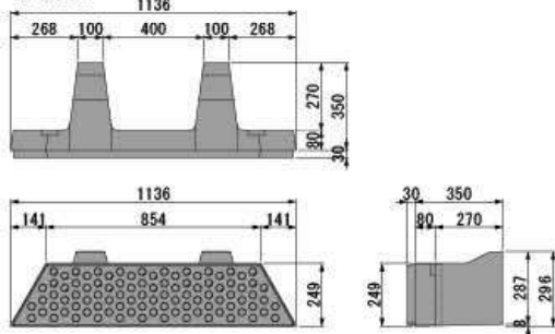
横半根石
