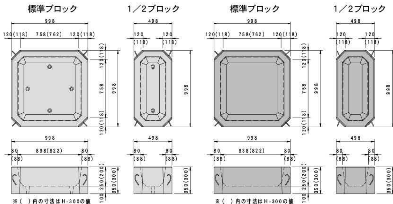
標準断面図
