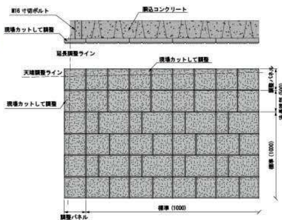
配列図
