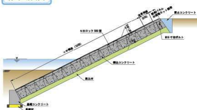
標準断面図
