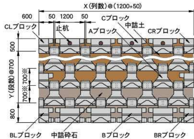
参考展開図
