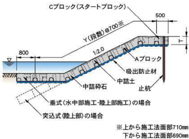
標準断面図
