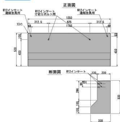
単体図
