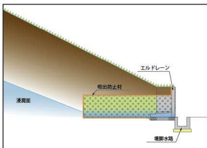
標準断面図
