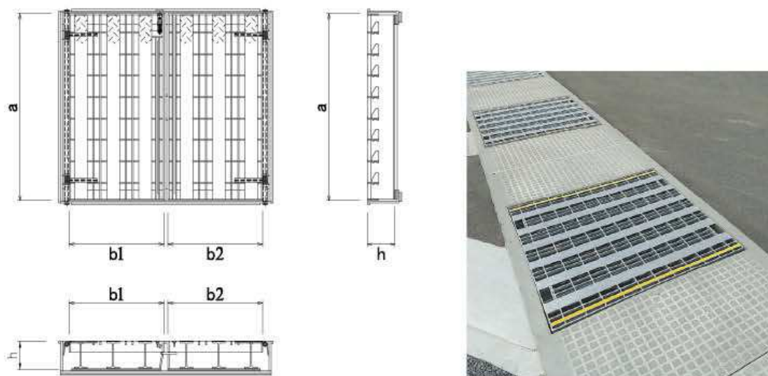
OS用エスカルゴグレーチング (T-25) 普通目
