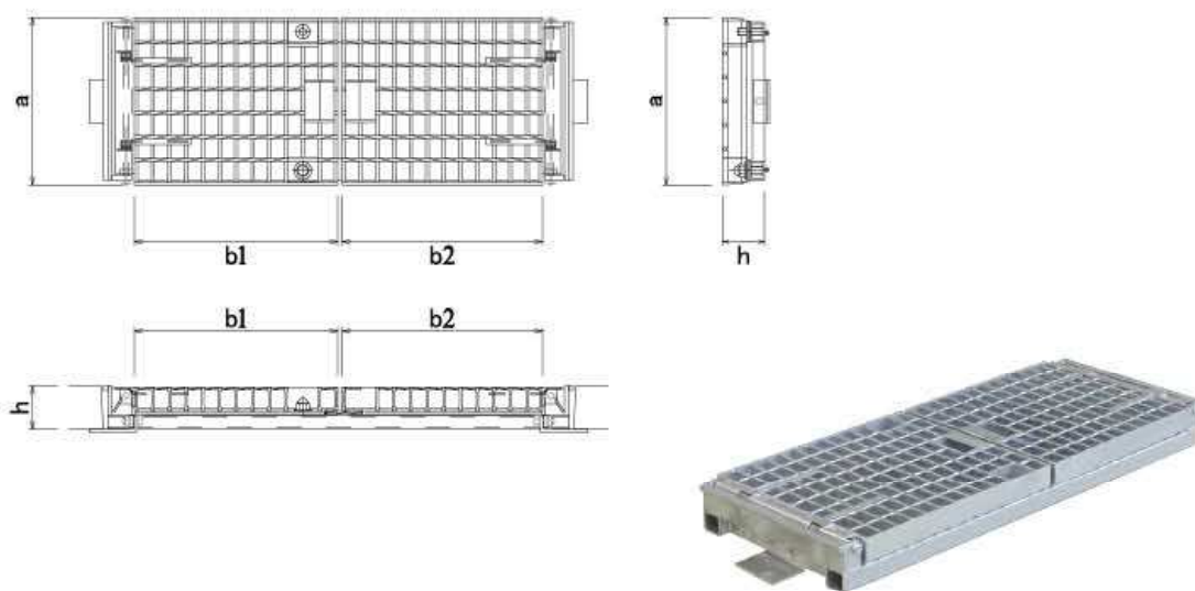
OS用Wロックエスカルゴグレーチング (T-25) 普通目
