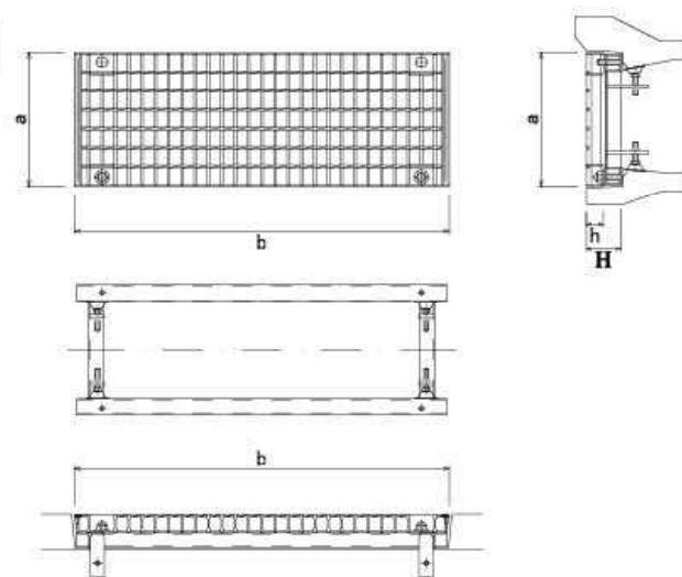
OS用ADJWロックグレーチング (T-25) 普通目
