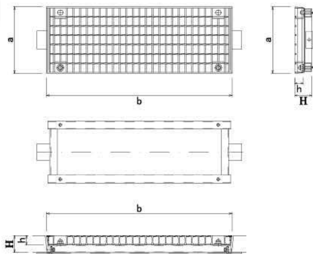
OS用Wロックグレーチング (T-25) 普通目
