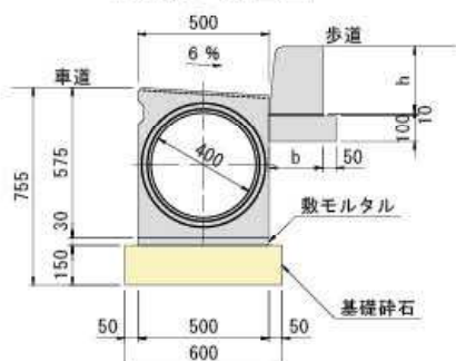
本体標準断面図
