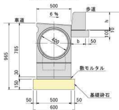
柵標準断面図
