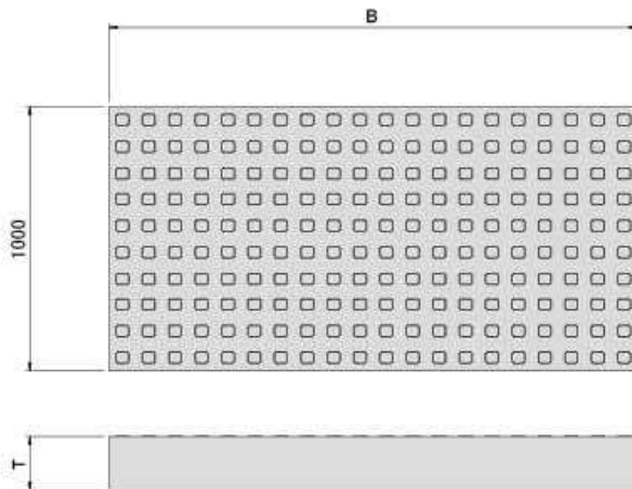
単体図
