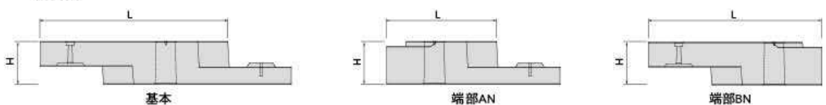
側面図
