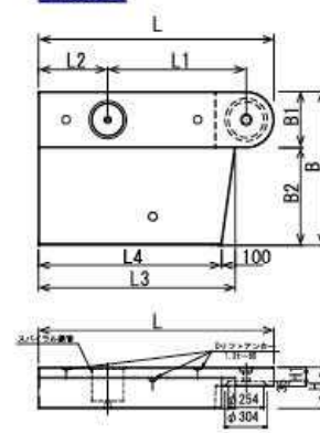
端部B
