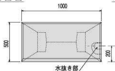
正面図
