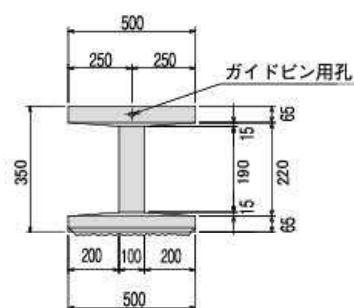
A-A断面図
