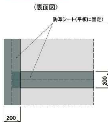
防草シート設置図
