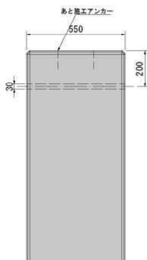
正面図
