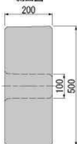
側面図
