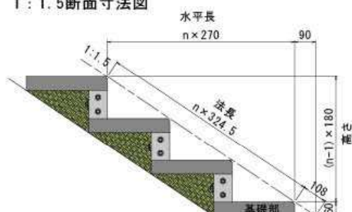
1 : 1.5断面寸法図
