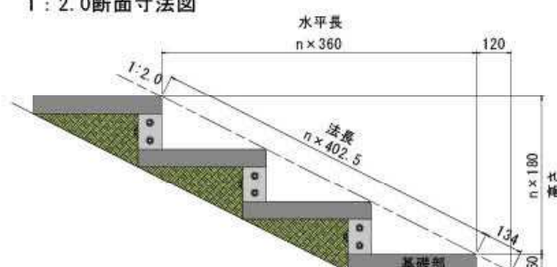
1 : 2.0断面寸法図
