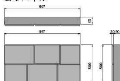
調整パネル
