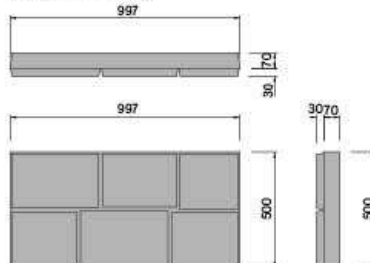
調整パネル
