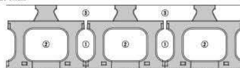
ブロック1個当たり数量表
