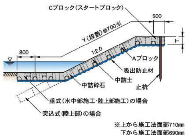
標準断面図
