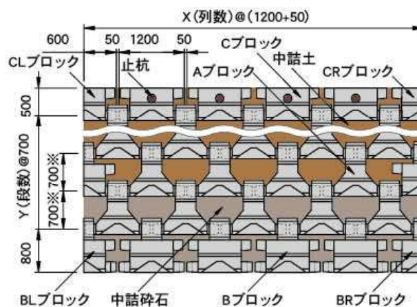
参考展開図
