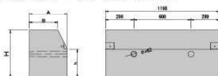
堤防法尻基礎ブロック400型、500型
