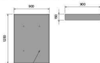
施工用インサート
