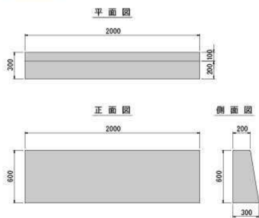
単体図
