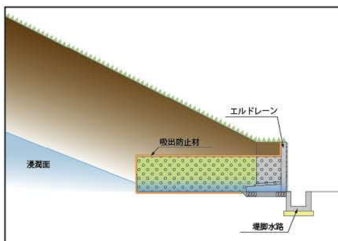
標準断面図
