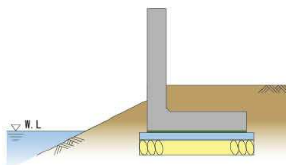
河川特殊堤
