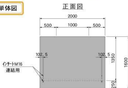
防潮堤
