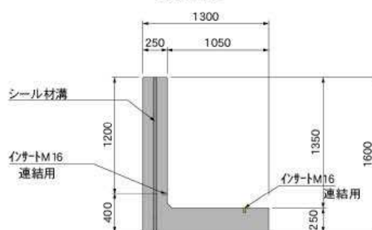
側面図
