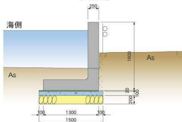
防潮堤
